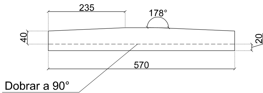
Peça B Chapa # 1/8" Quantidade: 02 Peças
