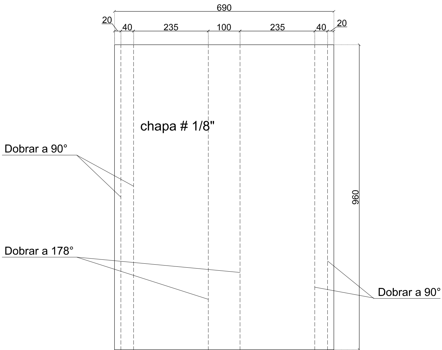
Peça A Chapa # 1/8" Quantidade: 01 Peça
